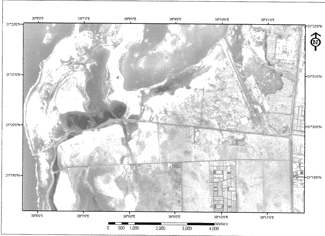
شكل (١) مرئية فضائية للقمر الصناعي أيكونوس لمنطقة الدراسة بدقة مكانية ١ متر التقطت عام ٢٠٠٥م.
