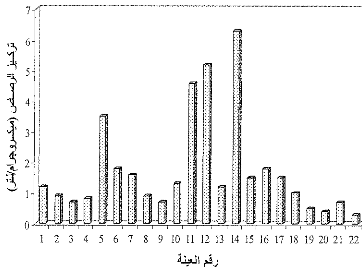
شكل (٧) توزيع عنصر الرصاص في المياه السطحية بمنطقة الدراسة.
