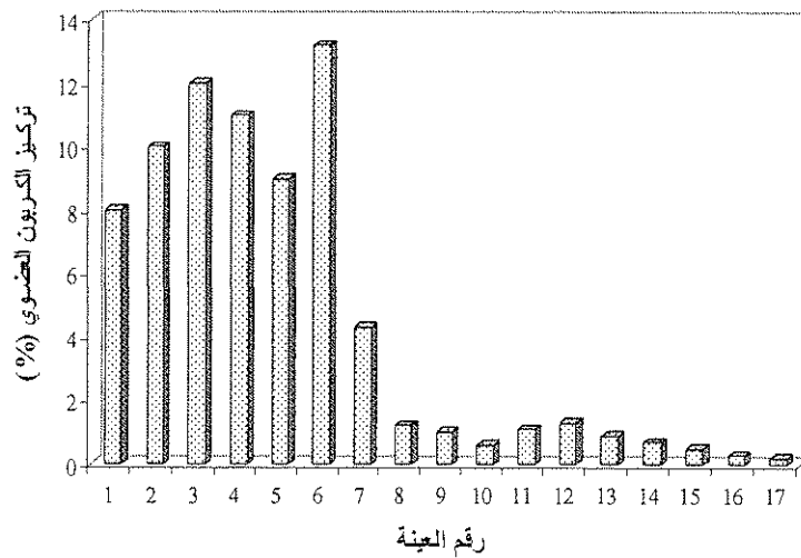
شكل (١٤) توزيع عنصر الكربون العضوي في الرواسب البحرية بمنطقة الدراسة.
