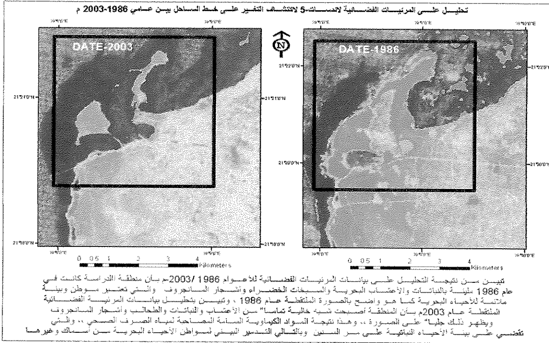
شكل (١٧) تحليل على المرئيات الفضائية لاندسات 5 لاكتشاف التغيير على خط الساحل بين عامي 1986-2003م.
