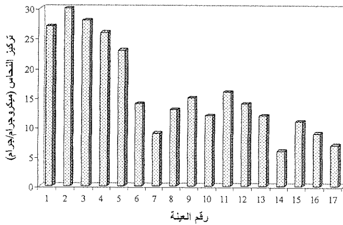
شكل (١١) توزيع عنصر النحاس في الرواسب البحرية بمنطقة الدراسة.
