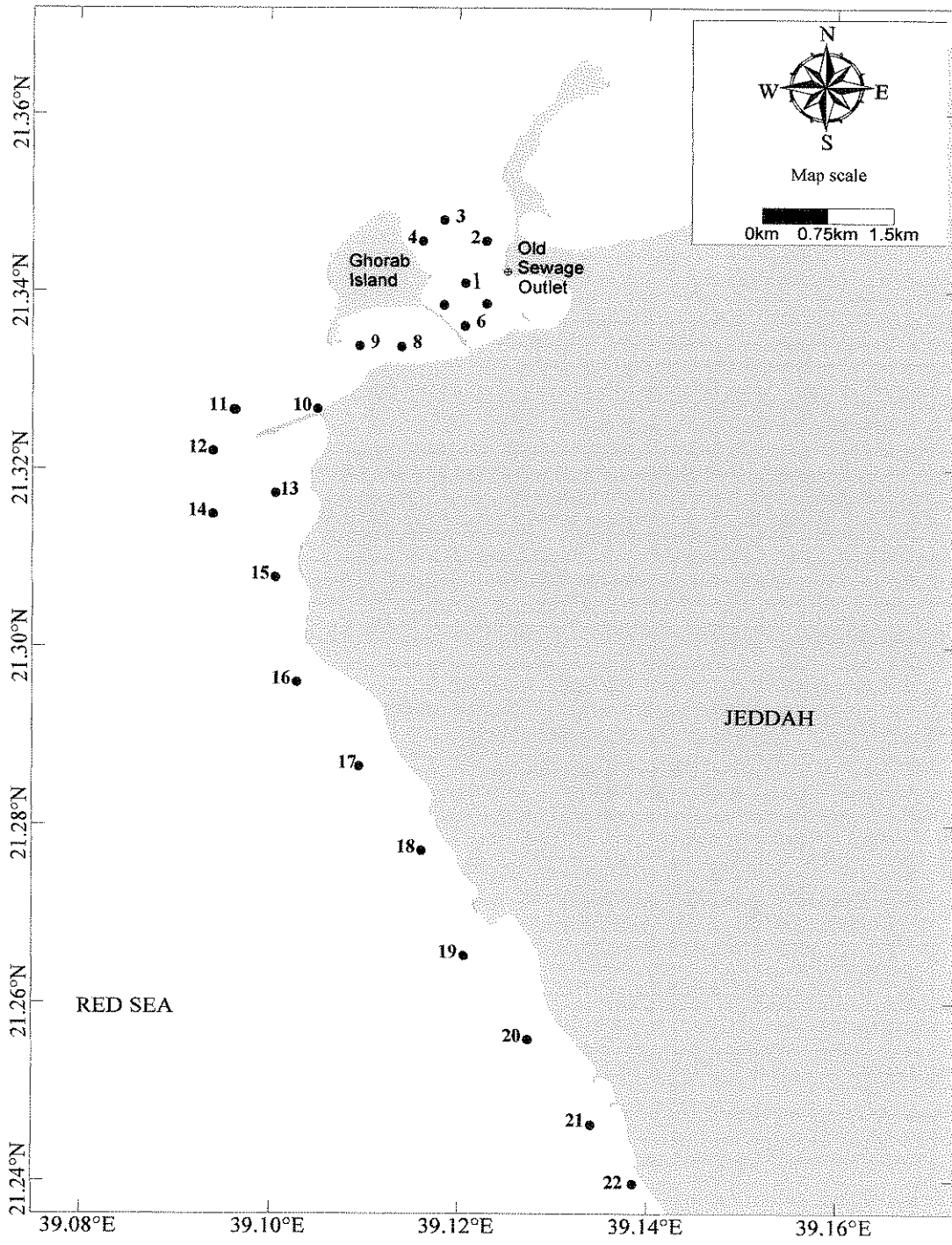
شكل (٢) مواقع جمع عينات المياه والرواسب في منطقة الدراسة.
