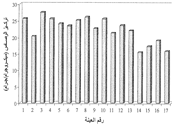
شكل (١٣) توزيع عنصر الزنك في الرواسب البحرية بمنطقة الدراسة.
