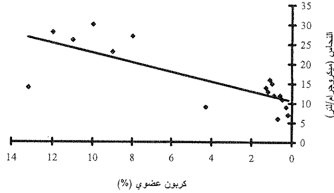
شكل (١٦) العلاقة بين النحاس والكربون العضوي.
